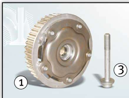
Fig. 1: Unitate de fazare dinspre admisie 427 1004 10 și șurub central 41301*
