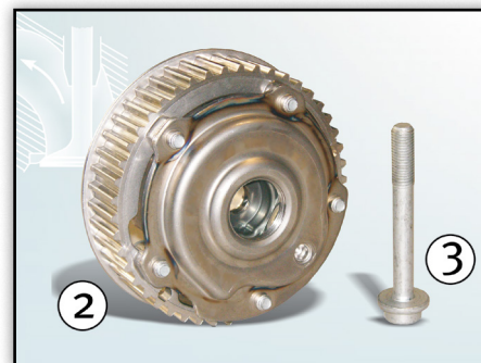
Fig. 2: Unitate de fazare dinspre evacuare 427 1005 10 și șurub central 41301*
