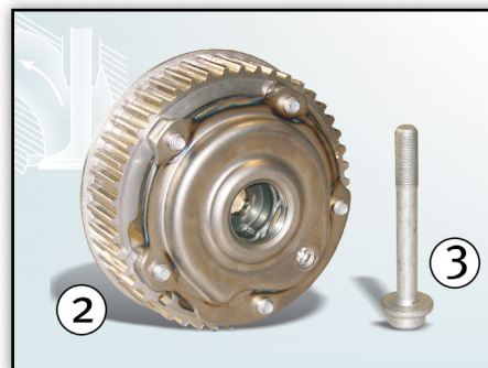
Снимка 2: Дефазатор на разпределителен вал от изпускателната страна 427 1005 10 и централен болт 41301*
