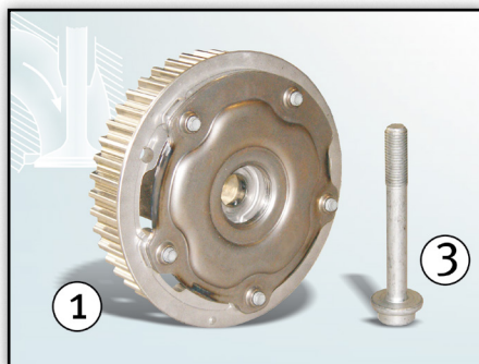
Снимка 1: Дефазатор на разпределителен вал от засмукващата страна 427 1004 10 и централен болт 41301*
