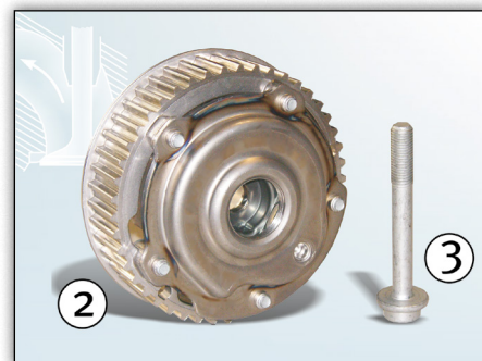
Figur 2: Kamakslens justering på udstødningsside 427 1005 10 og centralskrue 41301*
