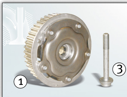
Εικόνα 1: Ρυθμιστής εκκεντροφόρου άξονα της πλευράς εισαγωγής 427 1004 10 και κεντρική βίδα 41301*
