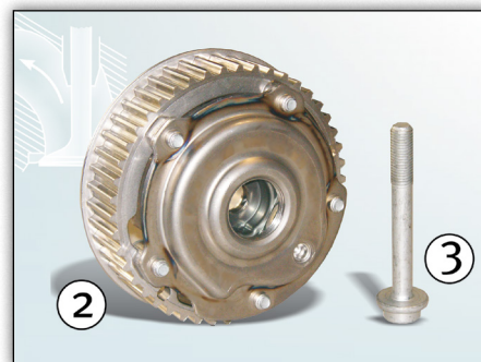
2. ábra: Kipufogó oldali vezérműtengely-állító 427 1005 10 és központi csavar 41301*
