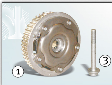
1. ábra: Szívóoldali vezérműtengely-állító 427 1004 10 és központi csavar 41301*
