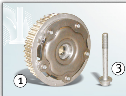
Bild 1: Kamaxeljustering insugsida 427 1004 10 och centralskruv 41301*
