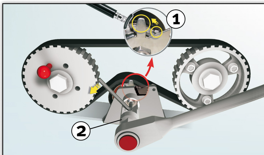
Fig. 1: Privire de ansamblu asupra sistemului, rolei și a instrumentului special de montare
