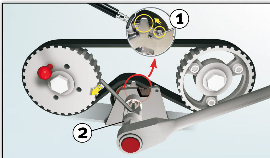
Снимка 1: Общ изглед на задвижването, на обтяжната ролка и на специализирания инструмент.
