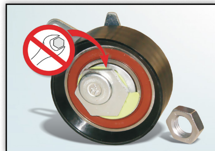
Снимка 2: Шестоъгълният фитинг на гърба на обтяжната ролка няма никаква функция.
