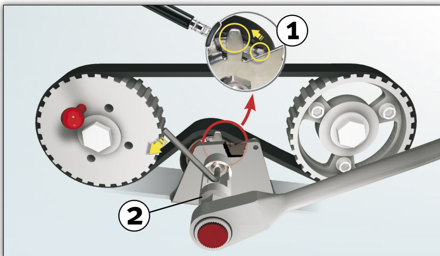
Obrázek 1: Přehled pohonu a polohy napínacích kladek a speciální nářadí
