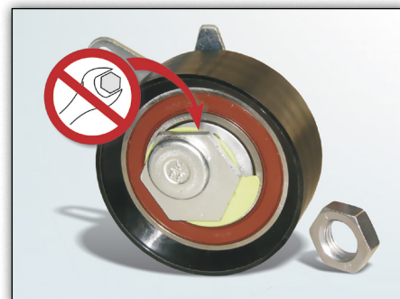
Obrázek 2: Šestihran na napínací kladce nemá žádnou funkci
