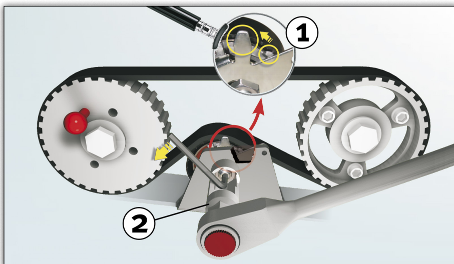
Εικόνα 1: Συνοπτική εικόνα μετάδοσης κίνησης και θέσης τοποθέτησης για τον εντωτήρα και ειδικό εργαλείο
