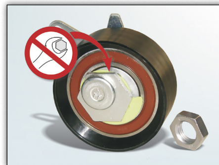
Εικόνα 2: Το εξάγωνο στον τεντωτήρα δεν έχει καμία λειτουργία
