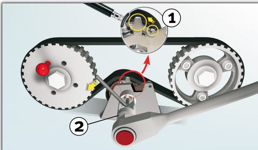
Kuva 1: Ruiskutuspumpun käyttöhihnajärjestelmä, hihnankiristin (tuotenro INA. 531 0573 30) sekä erikoistyökalu
