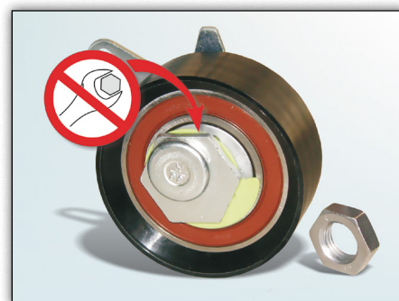
Kuva 2: Kiristimen takana olevalla levyllä ei ole toiminnallista merkitystä.
