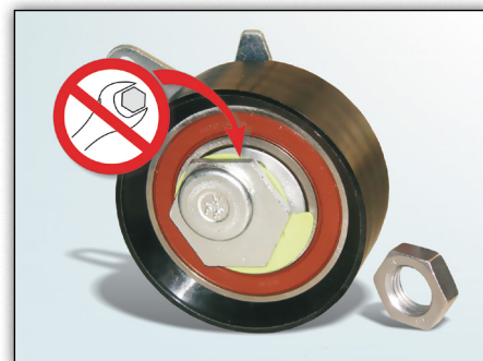
2. ábra: A feszítőgörgőn lévő hatlapnak nincs funkciója
