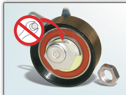
Bild 2: Sexhörningen på spännrullen saknar funktion
