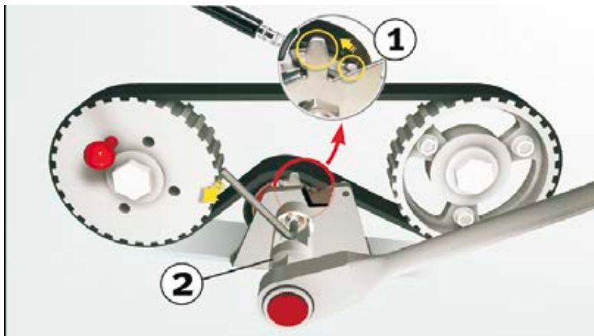
Рис. 1: Регулятор фаз газораспределения на впуск 427 1004 10 и центральный болт 41301*
