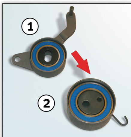
Fig. 1: Rolă întinzătoare înlocuită 531 0166 20 (1) și modelul înlocuitor 531 0819 10 (2)
