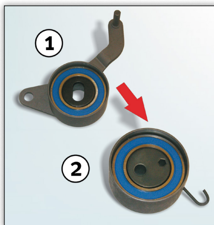
Снимка 1: Заменена обтяжна ролка 531 0166 20 (1) и нейният приемник 531 0819 10 (2)
