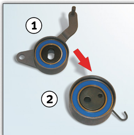
Figur 1: Erstattet strammerulle 531 0166 20 (1) og dens efterfølger 531 0819 10 (2)
