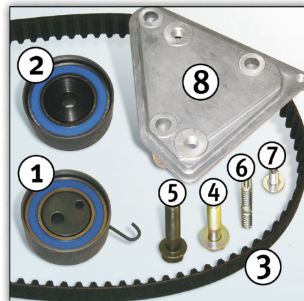
Εικόνα 2: Περιεχόμενο συσκευασίας 530 0492 10
