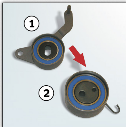
Εικόνα 1: Αντικατεστημένος τεντωτήρας 531 0166 20 (1). Νέος σχεδιασμός με κωδικό 531 0819 10 (2)
