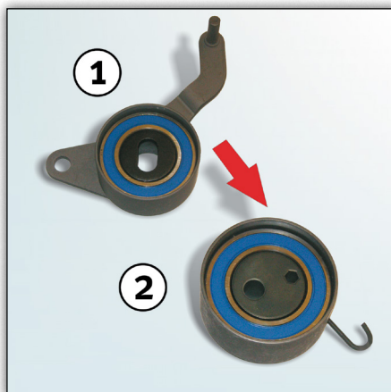
Kuva 1: 1. Korvattu hihnankiristin 531 0166 20 2. Uusi hihnankiristin 531 0819 10
