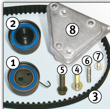
Bild 2: Innehåll i förpackning 530 0492 10
