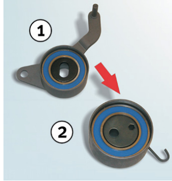
Resim 1: Eski gergi rulmanı 531 0166 20 (1) ve yeni gergi rulmanı 531 0819 10 (2)
