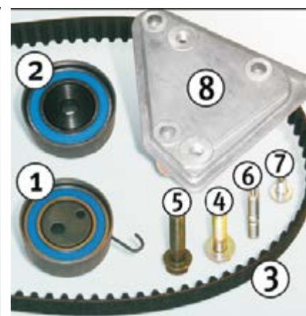
Рис. 2: Состав упаковки: 530 0492 10
