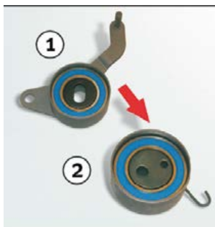
Рис. 1: Замена натяжного ролика 531 0166 20 (1) на 531 0819 10 (2)
