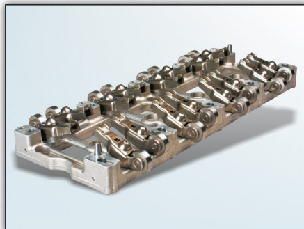
Obrázek 1: Lůžko vahadel 423 0061 10
