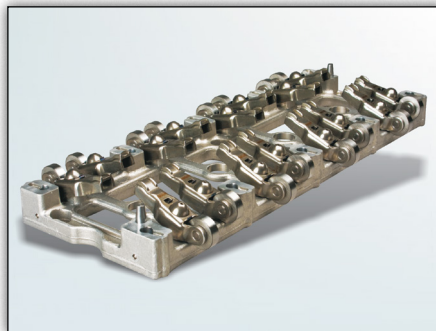
Εικόνα 1: Βάση ζυγώθρου 423 0061 10
