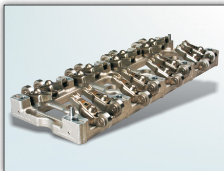
Kuva 1: Keinuvivun laakerin teline 423 0061 10
