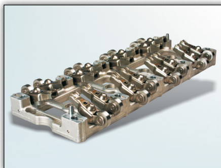
1. ábra: Himbaállvány 423 0061 10
