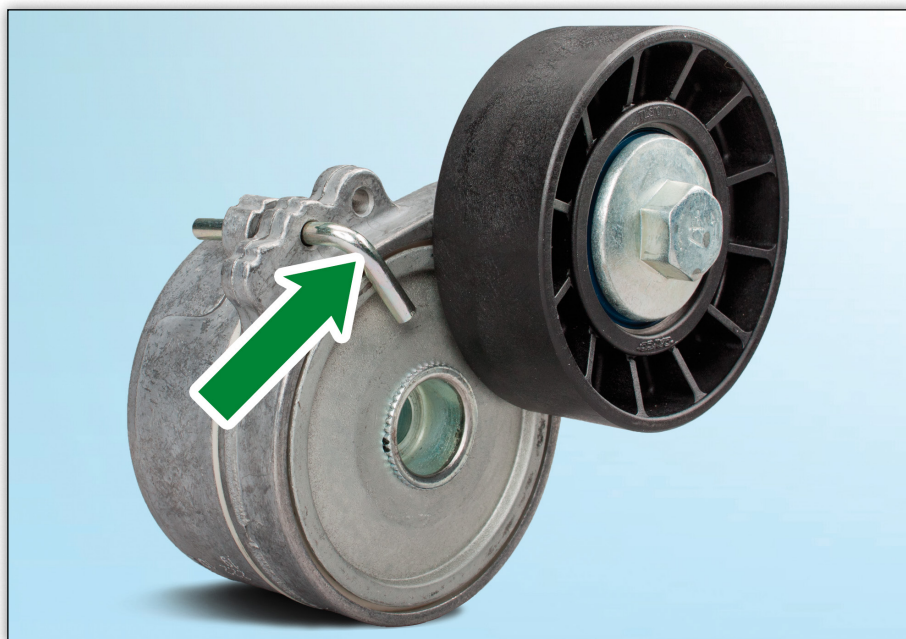
Снимка 1: 534 0110 20 — обтягащо рамо със застопоряващ щифт на INA
