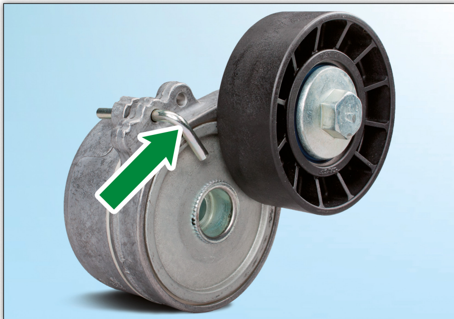
Obrázek 1: 534 0110 20 – INA-napínací jednotka s pojistným kolíkem
