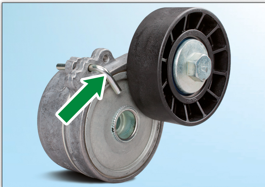
Figur 1: 534 0110 20 - INA-strammearm med sikkerhedsnål
