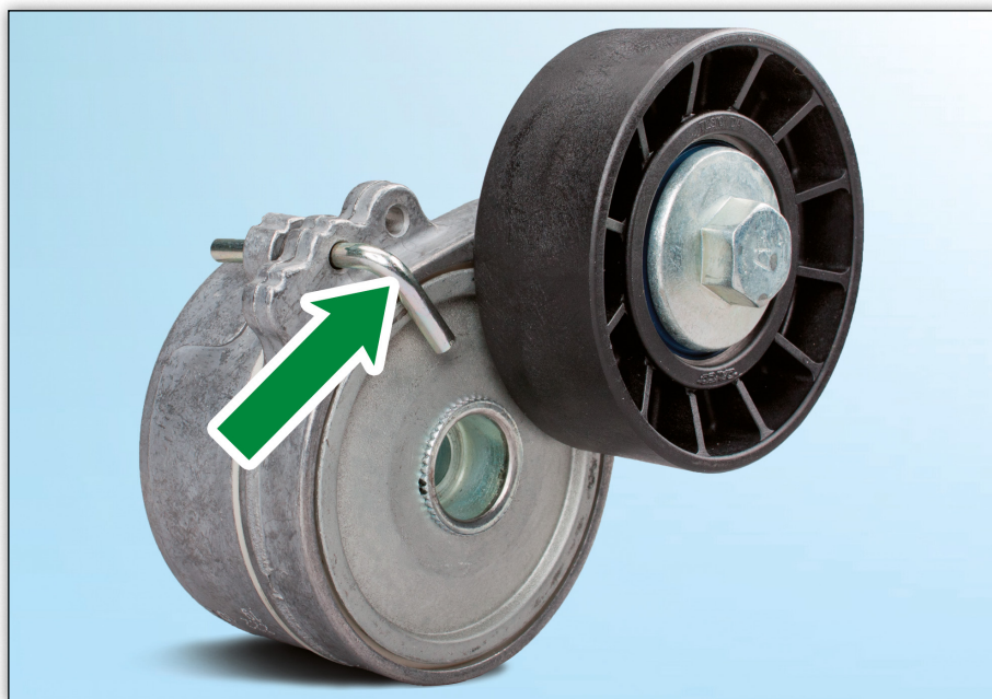
Εικόνα 1: 534 0110 20 - Βραχίονας τάνυσης INA με πείρο ασφάλισης.
