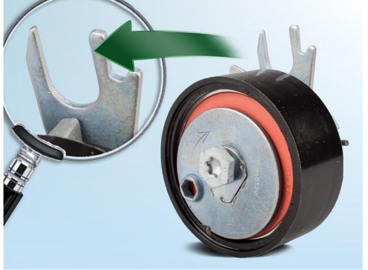
Resim 1: 531 0317 10 referanslı montaj plakası kelepçesi bulunan gergi rulmanı
