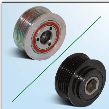
Bild 1: Hittillsvarande kända utförande Toyota (silver), Kia/Hyundai (svart)
