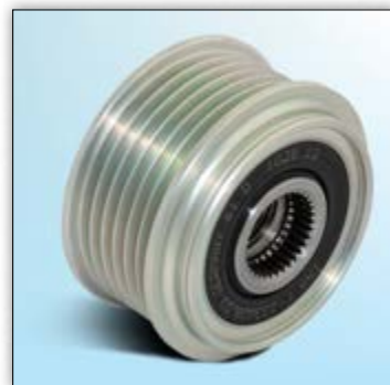
Рисунок 2: Новая конструкция
