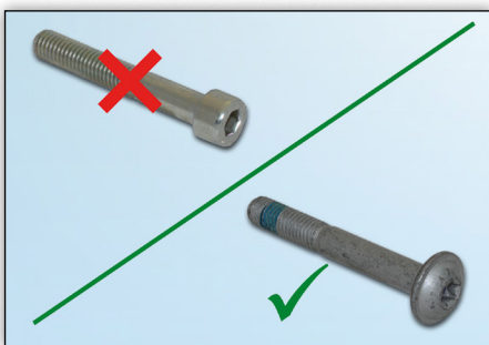
Снимка 3: болт
