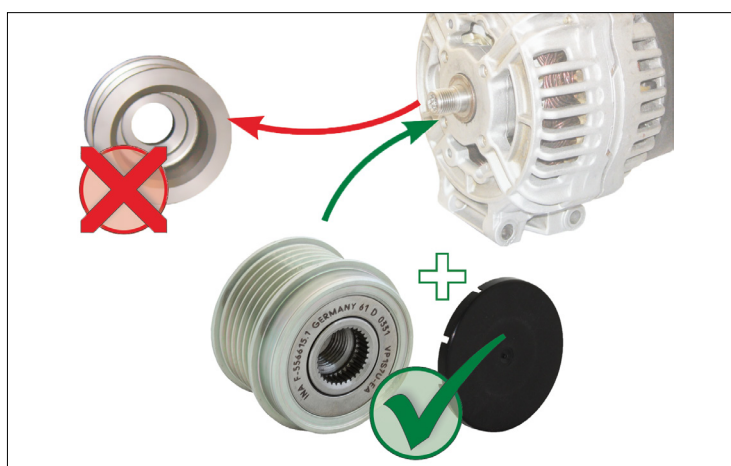
Figur 1: Udskiftning af en fast remskive for et friløbshjul til generator
