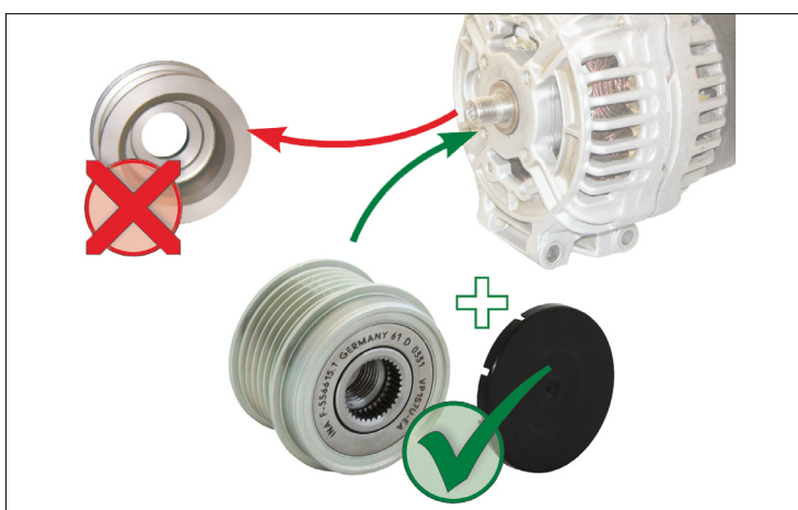
Kuva 1: Kiinteän hihnapyörän vaihto laturin vapaapyörään
