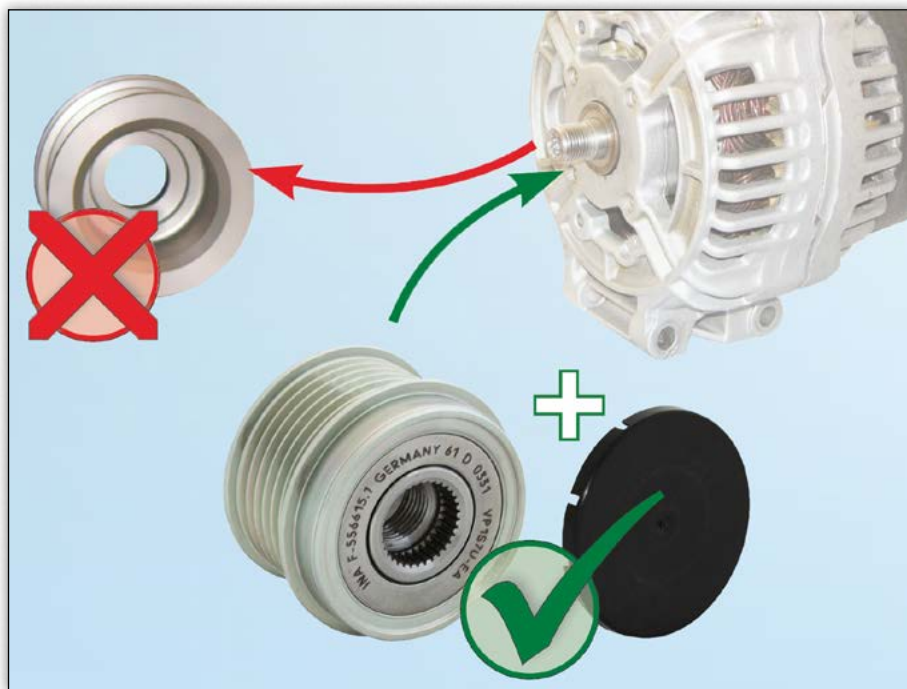
1. ábra: Váltás a merev szíjtárcsáról a generátor-szabadonfutóra
