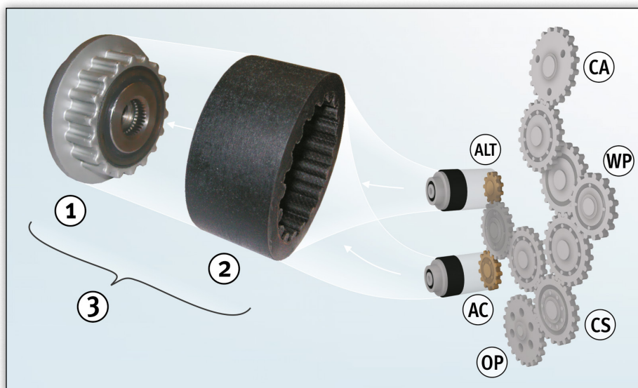
Obrázek 1: Alternátorová volnoběžka s flexibilní spojovací objímkou a pohonem koly s čelním ozubením
