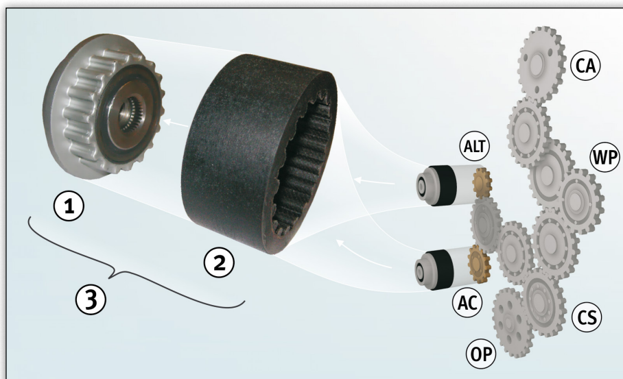
Figur 1: Friløbshjul til generator med en elastisk forbindelsesmuffe og drivsystemet med forreste tandhjul
