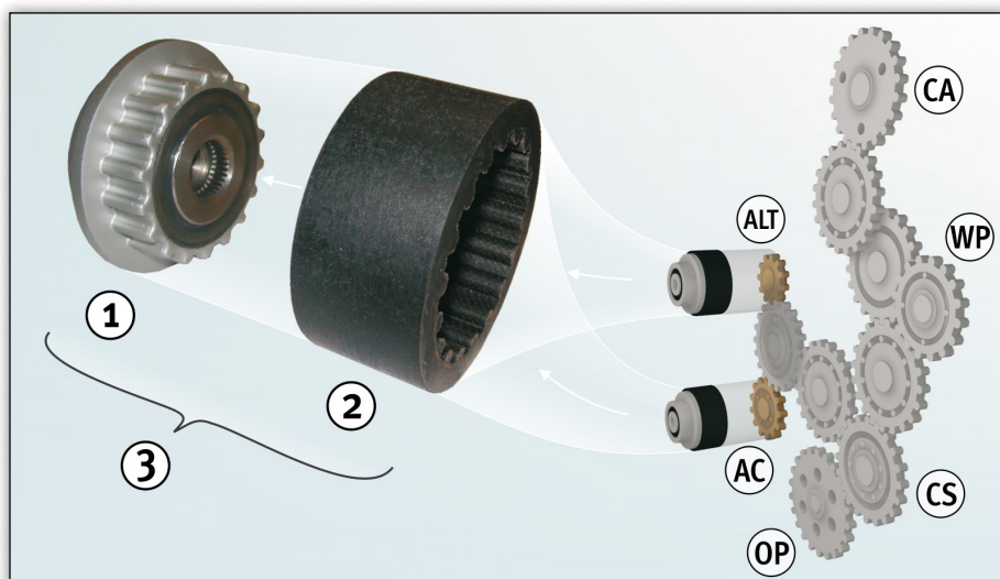
Εικόνα 1: Τροχαλία δυνάμο με κασάνια με εύκαμπο χιτώνιο σύνδεσης και γρανάζι με ευθεία οδόντωση
