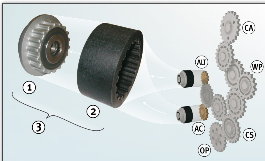
1. ábra: Generátor-szabadonfutó rugalmas kuplungaggal és homlokkerék-meghajtással
