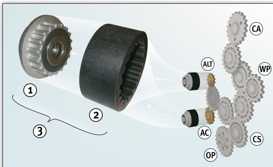
Bild 1: Generatorfrinav med flexibel kopplingsmuff och drivning genom främre kugghjul.
