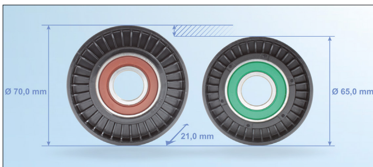
Imaginea 2: Fulia defletoare 532 0404 30 pentru vehiculele cu motor pe benzină (stânga) și fulia defletoare 532 0406 30 pentru vehiculele cu motor diesel (pe motorină) (dreapta)
