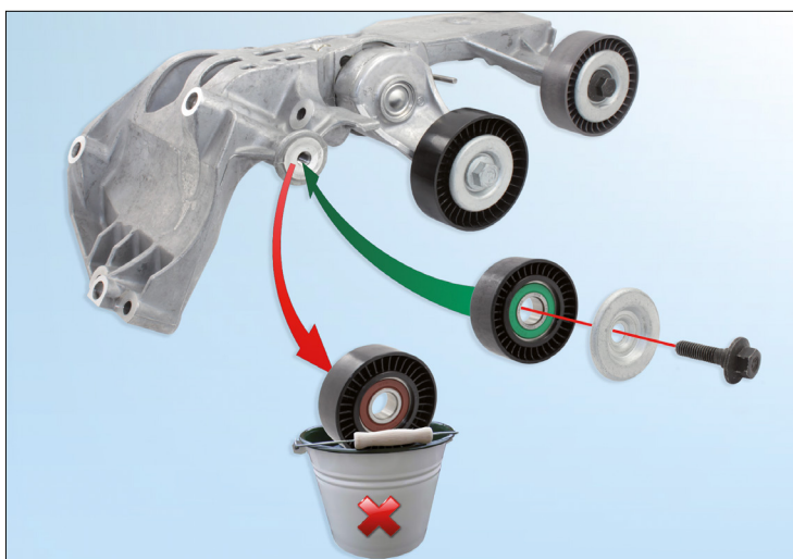
Imaginea 1: Unitate întinzătoare 534 0243 10
