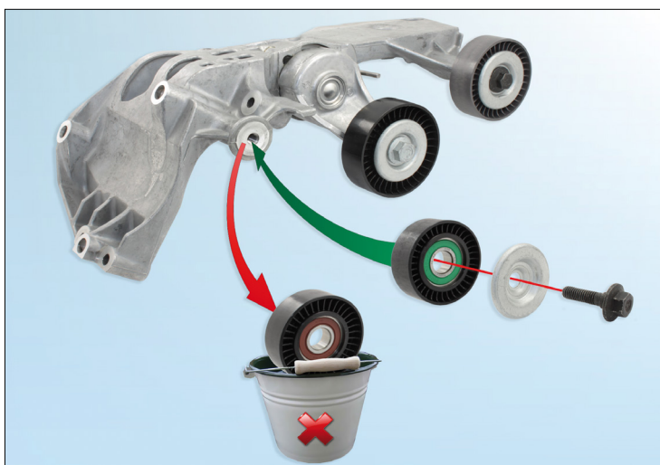
Снимка 1: Обтяжен елемент 534 0243 10
