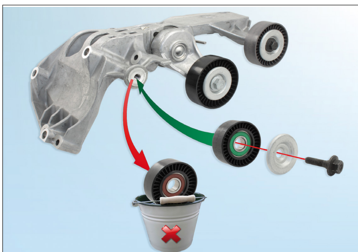
Obrázek 1: Napínací jednotka 534 0243 10
