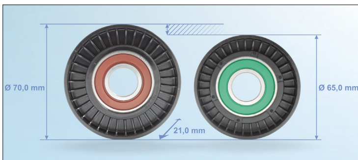
Obrázek 2: Vodicí kladka 532 0404 30 pro vozidla se zážehovým motorem (vlevo) a vodicí kladka 532 0406 30 pro vozidla se vznětovým motorem (vpravo)
