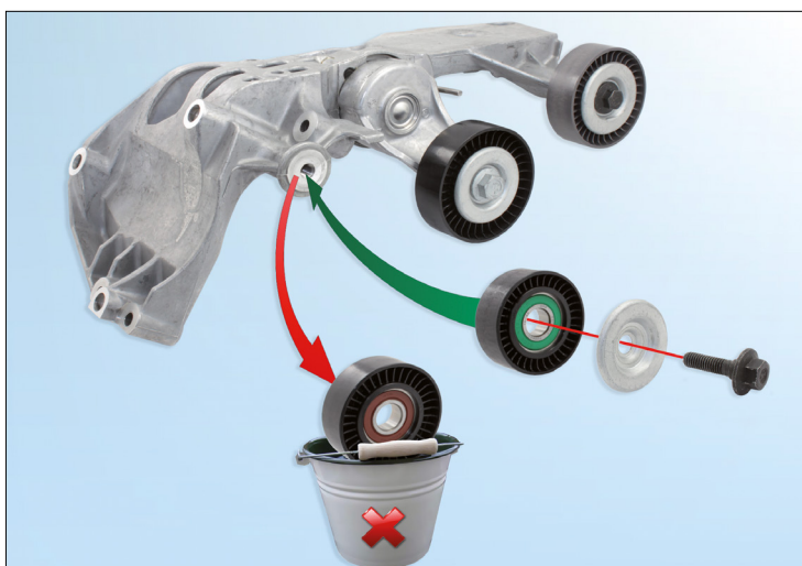
Figur 1: Strammeenhed 534 0243 10
