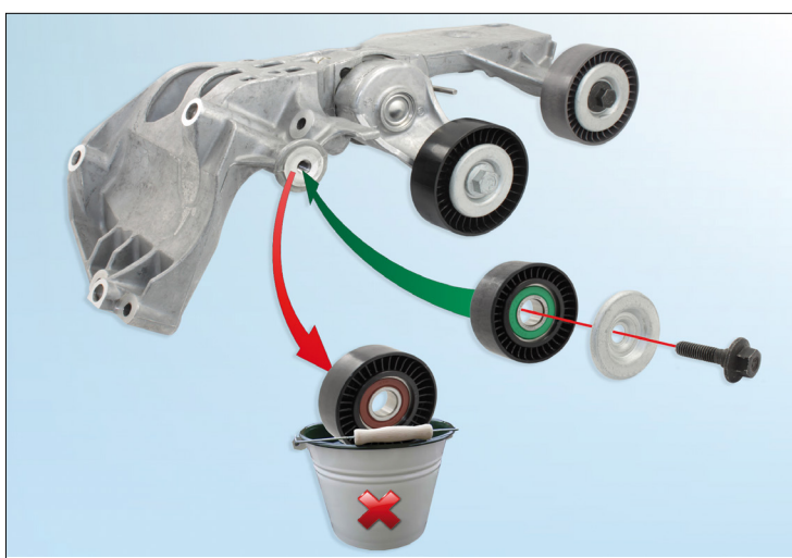
Εικόνα 1: μονάδα τάνυσης 534 0243 10
