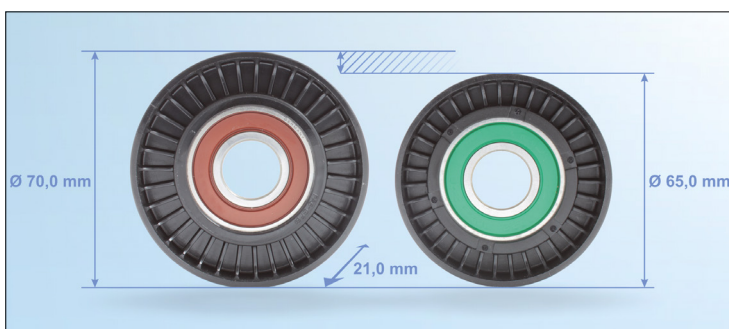
Kuva 2: Ohjainpyörä 532 0404 30 ottomoottorilla varustettuihin autoihin (vasemmalla) ja ohjainpyörä 532 0406 30 dieselmoottorilla varustettuihin autoihin (oikealla)
