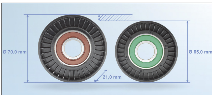
Slika 2: Remenica klizača 532 0404 30 za benzinske motore (lijevo) i remenica klizača 532 0406 30 za diesel motore (desno).
