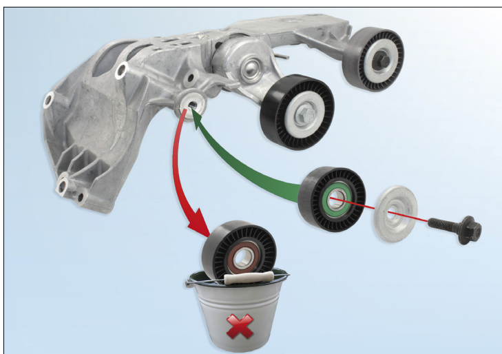
Slika 1: Sklop nosača - kataloški broj 534 0243 10
