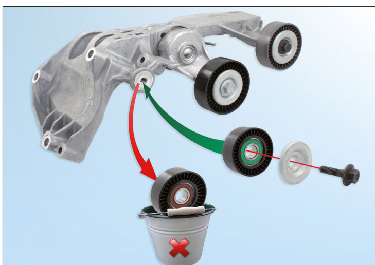
1. ábra: Feszítőegység 534 0243 10
